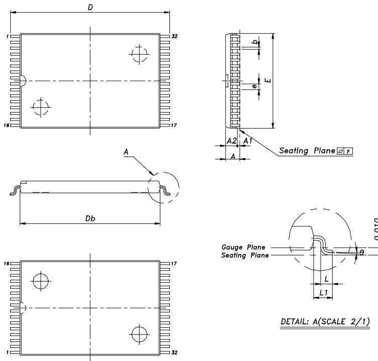
STSOP-32
