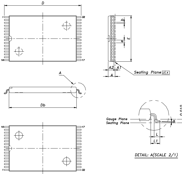
STSOP-32
